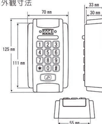
■外観寸法
